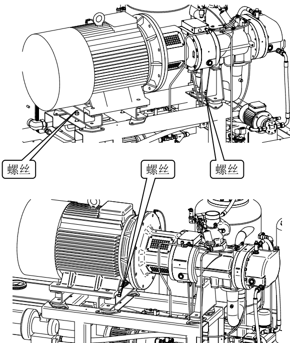
图 5-4 搬运固定螺丝
