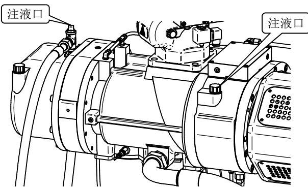
图 6-2 机体注液口
