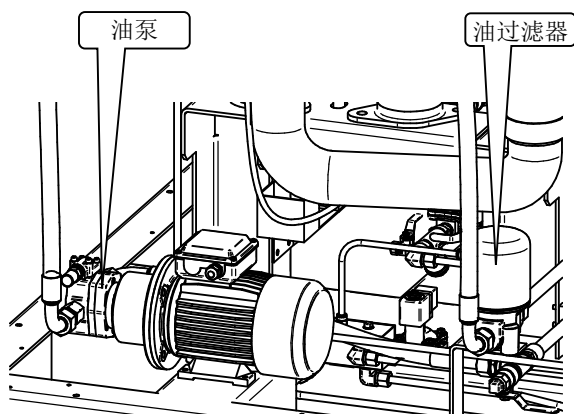
图 1-13 油泵与油过滤器
