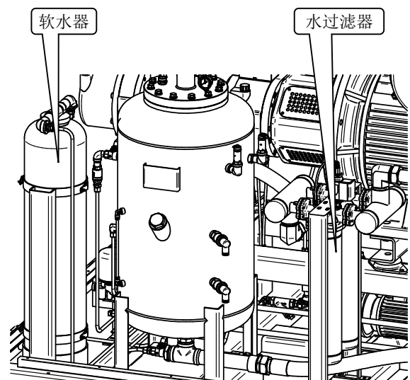
图 1-11 水过滤器与软水器
