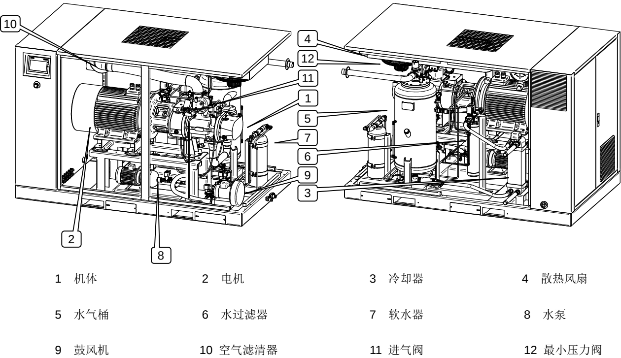
图 1-2 SWV30-37W 喷水无油螺杆式空压机内部构造
