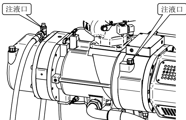
图 5-5 机体注液口
