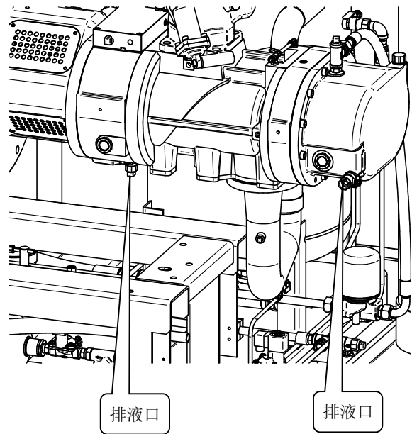
图 6-4 机体排液口
