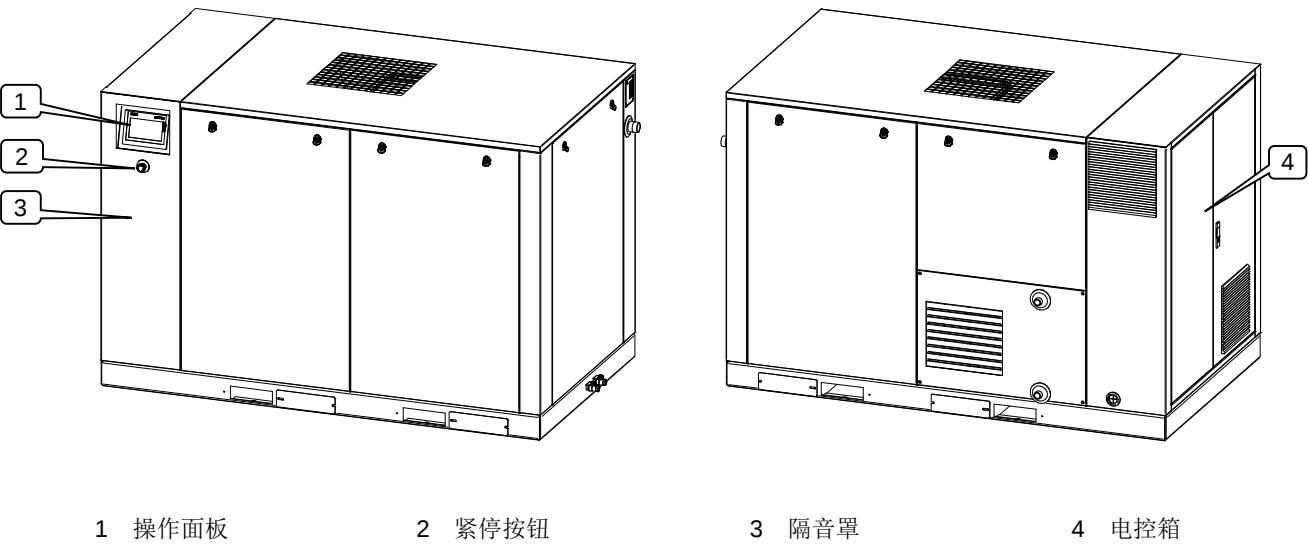
图 1-1 SWV30-37W 喷水无油螺杆式空压机外观
