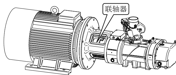
图 1-6 机体驱动
