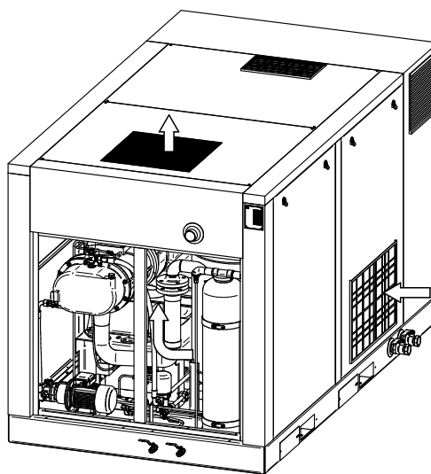
图 1-14 空压机冷却流场
