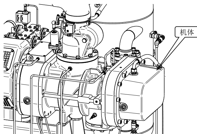
图 1-8 机体
