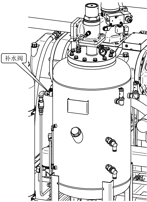
图 6-3 水气桶补水阀
