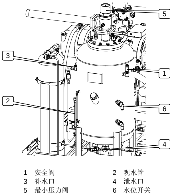
图 1-9 水气桶
