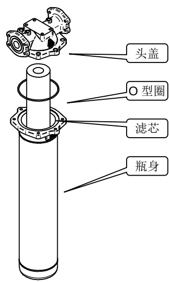
图 6-5 水过滤器
