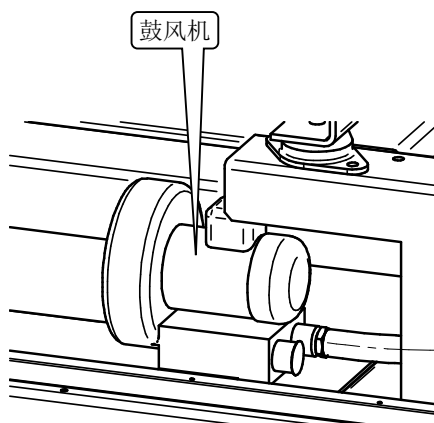
图 1-12 鼓风机
