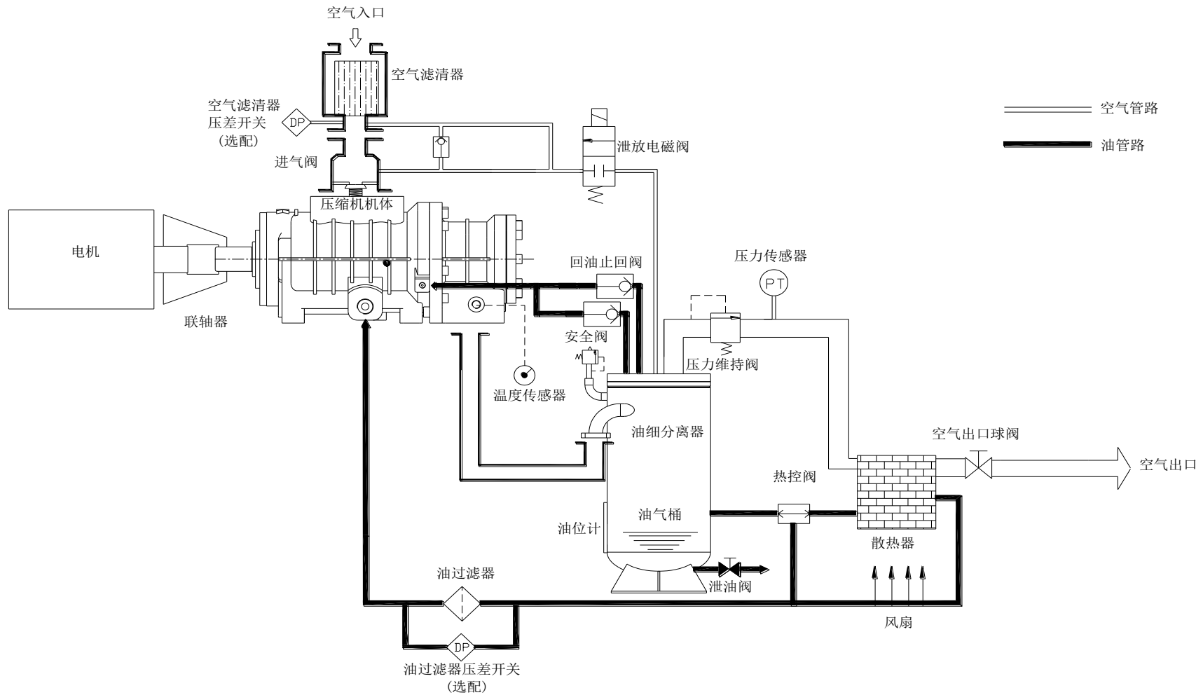
SLV30~185A 系统流程图
