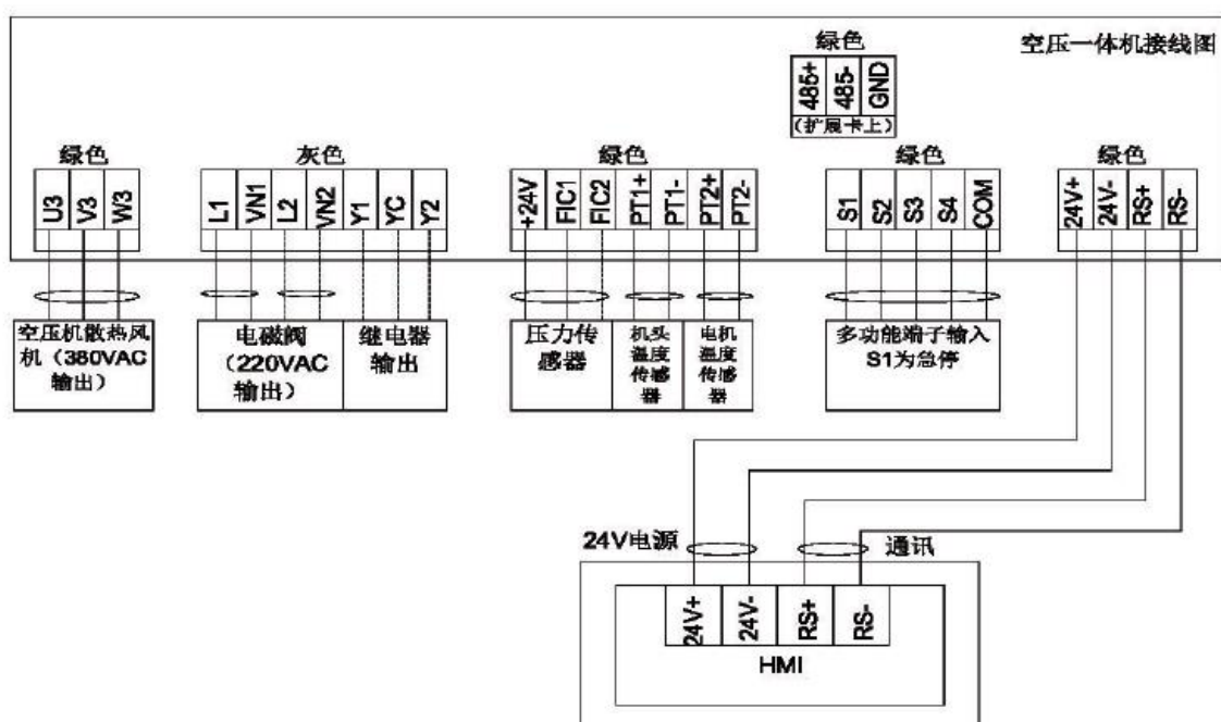
SAV04-37 原理图
