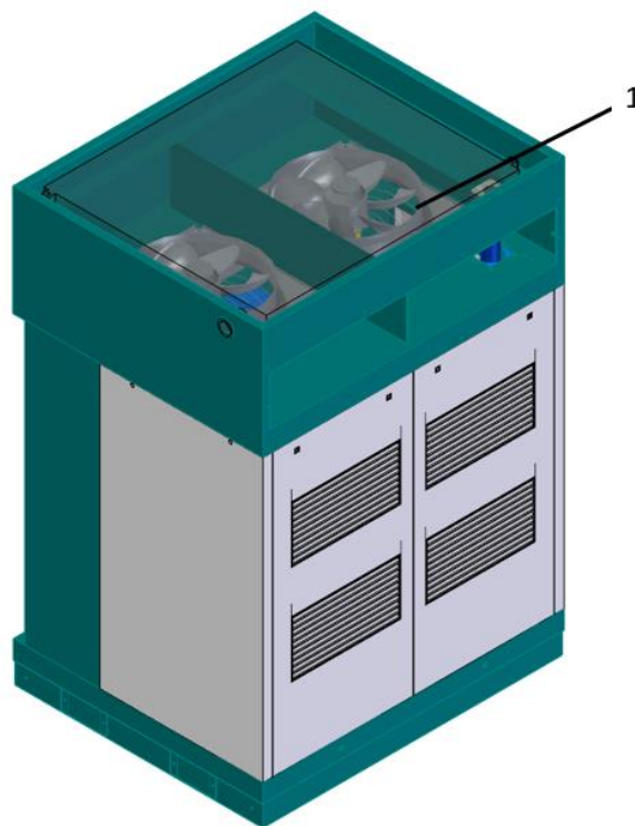
图 13: 冷却风扇
