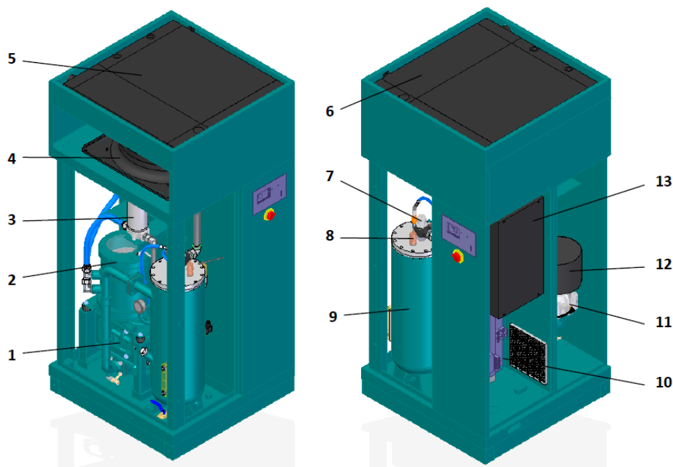
图 2: 37 - 75 kW螺杆空压机, 配备一体式电机、变频器
