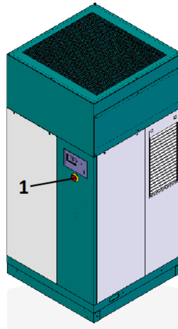
图 16：螺杆式空压机37–75 kW的紧急按钮(1)
