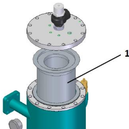
图 9：油细分离器
