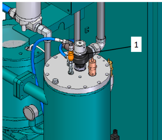
图 10：压力维持阀
