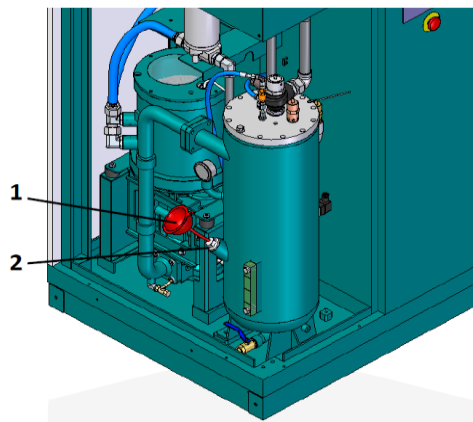
图 32 : 加油口
