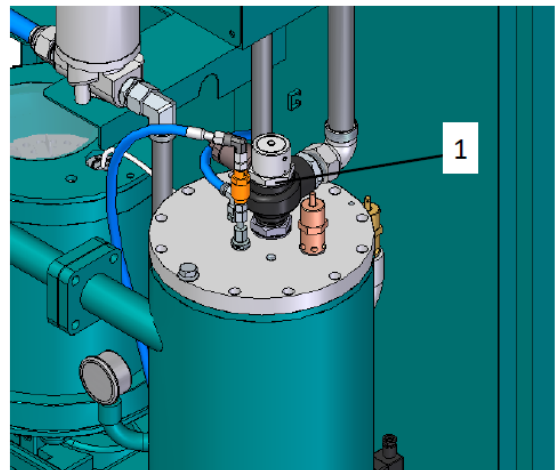
图 10：压力维持阀
