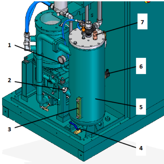
图 8：含安全阀的油气桶
