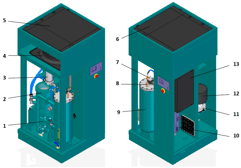
图 2： 06–37 kW螺杆空压机，配备一体式电机、变频器
