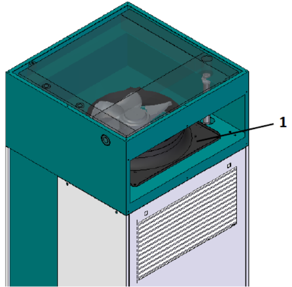
图 13: 冷却风扇
