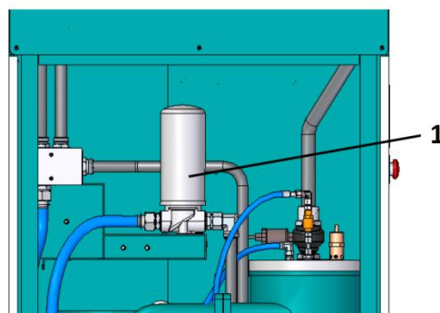
图 38：油过滤器
