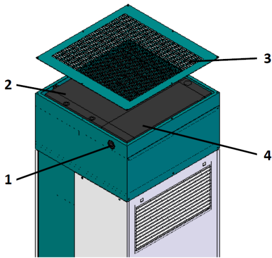
图 11: 冷却器
