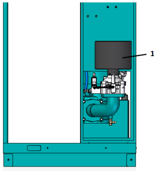
图 5: 进气过滤器
