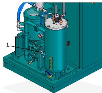
图 35 : 加油口塞头
