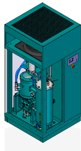
图 23：直联传动螺杆式空压机
