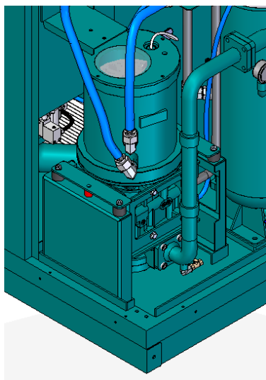
图 4: 一体式直联螺杆式空压机
