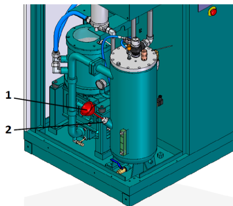
图 37：加油口
