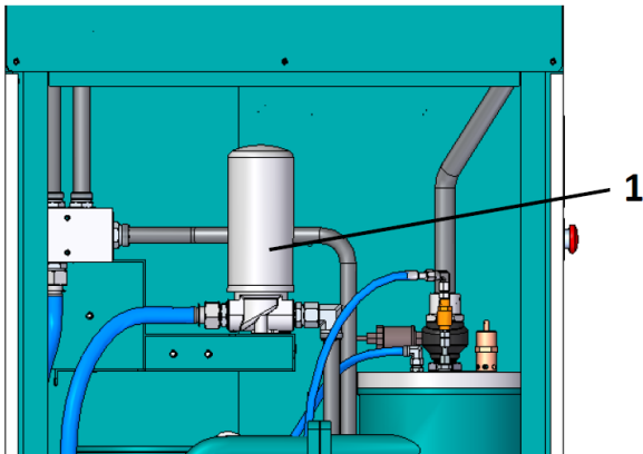
图 12: 油过滤器
