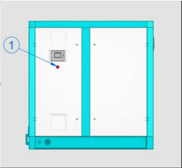
图 1：螺杆式空压机90-250kW 紧停按钮位置
