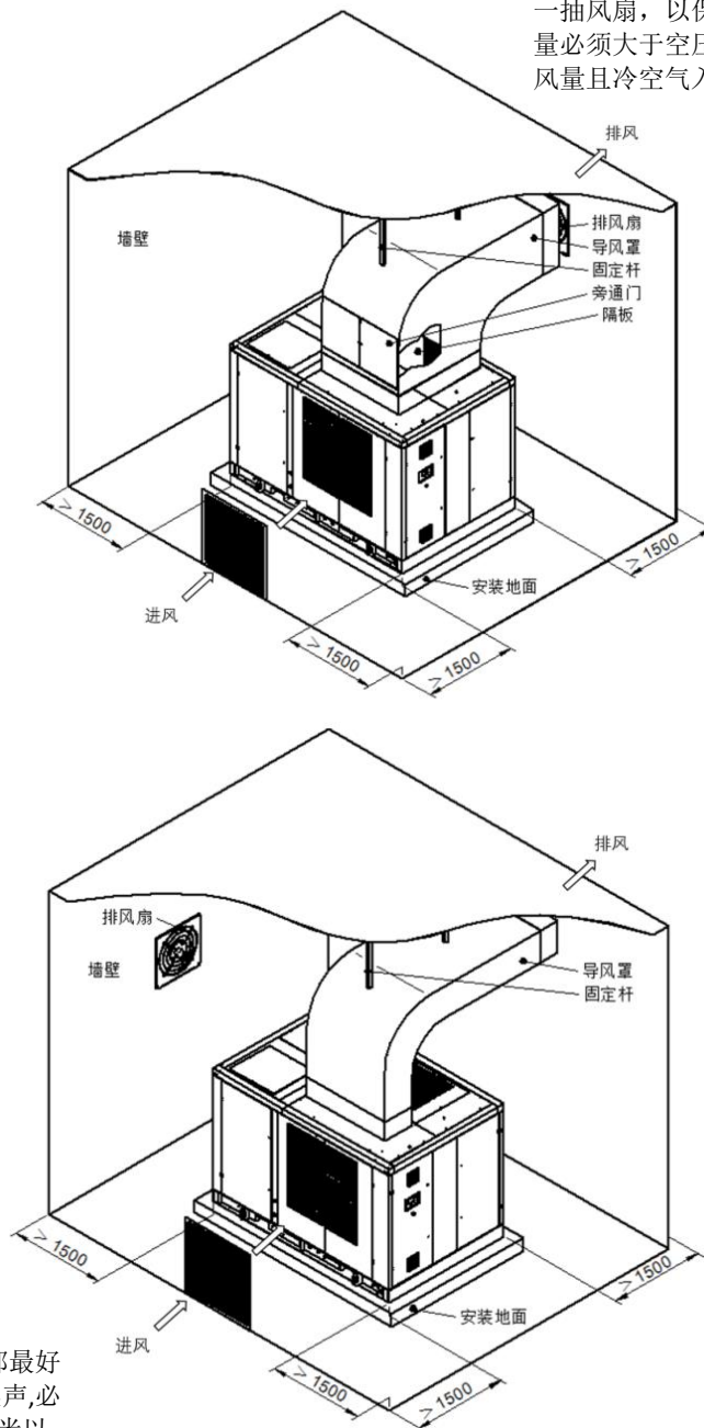
图 6：安装空间示意图
