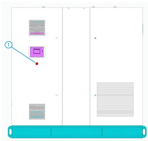
图 1：螺杆式空压机55-200kW 紧停按钮位置
