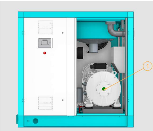
图 4：螺杆式空压机55-200kW，电机运转方向位置
