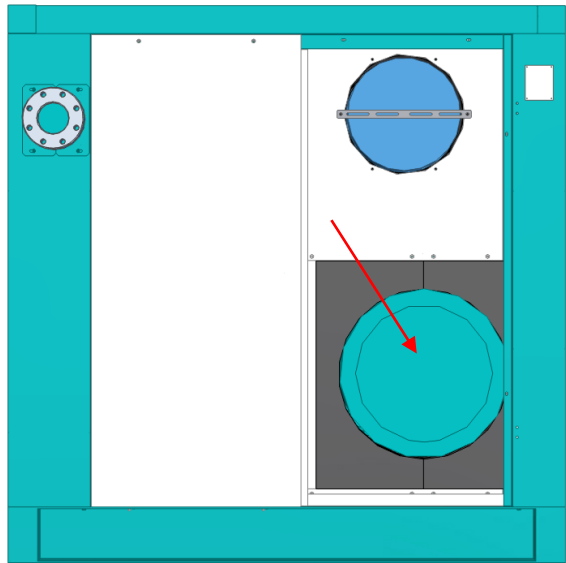
图 5：螺杆式空压机90-250kW，电机运转方向位置
